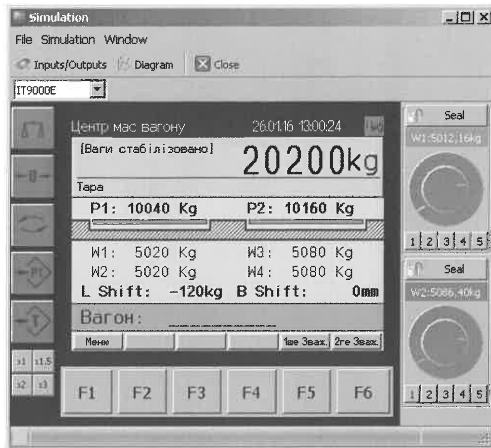
Рис. 1: Схема ваг
